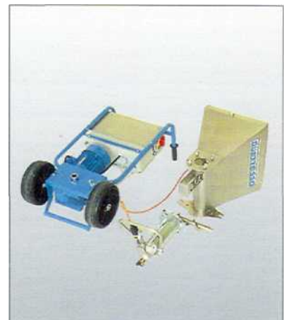
Module der S 30: Antrieb, Behälter und Pumpe
