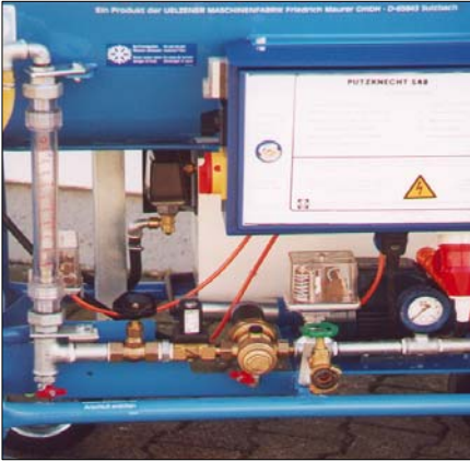
Kompakt-Wasserarmatur mit integriertem Niederdruckminderer.
