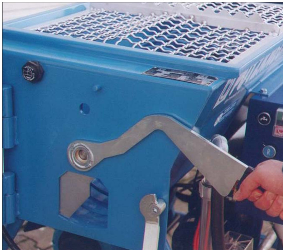
Verbesserter Schieber zwischen Trockenbehälter und Mischkammer. Voll geladnen mit trocken Material kann die Arbeit unterbrochen werden.
